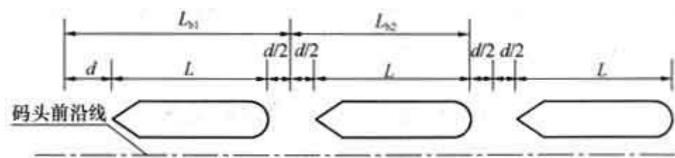
图 4.4.2-2 多个泊位长度
